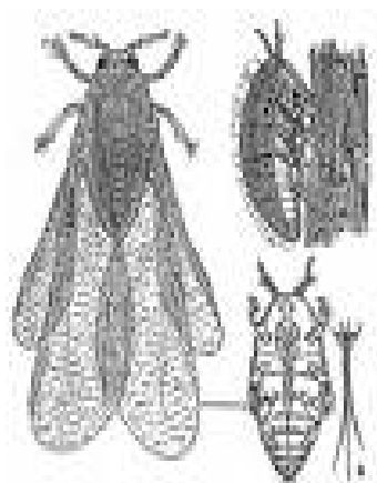
Εικόνα 20. Phylloxera vitifoliae
